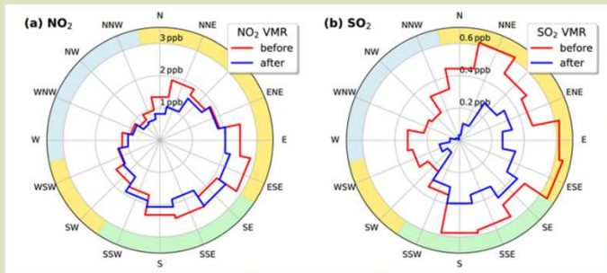
Messungen von NO 2 und SO 2 auf Neuwerk (abhängig von der Windrichtung) vor und nach dem Inkrafttreten neuer Richtlinien für den Schwefelgehalt in Schiffstreibstoffen Anfang 2015
