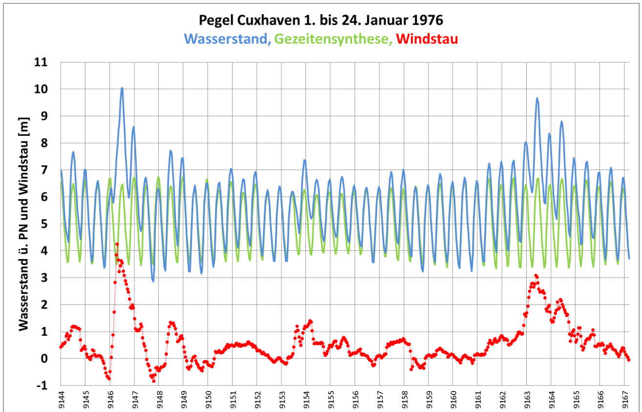
Wasserstandsganglinien am Pegel Cuxhaven-Steubenhöft im Januar 1976
