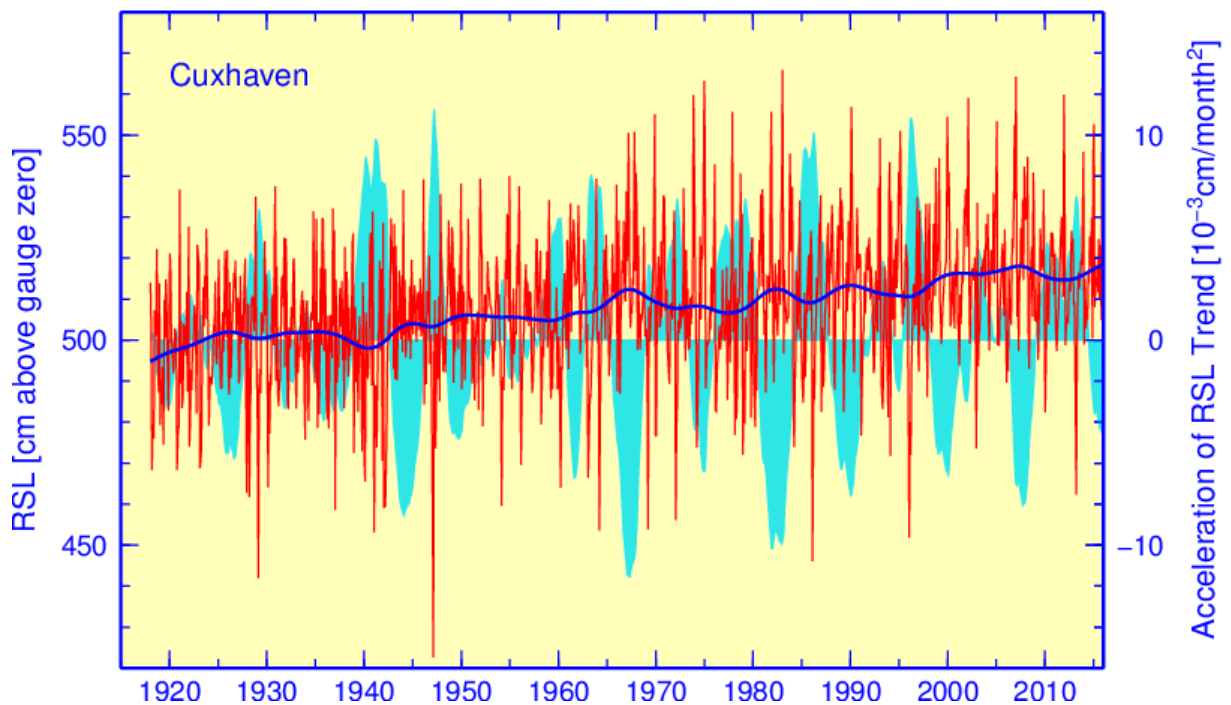
Meeresspiegelanstieg am Pegel Cuxhaven-Steubenhöft, abgeleitet aus stündlichen Beobachtungen des Wasserstandes.
